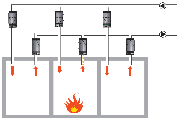
6.3 EKO-BSVF monterat utanför brandrummet
